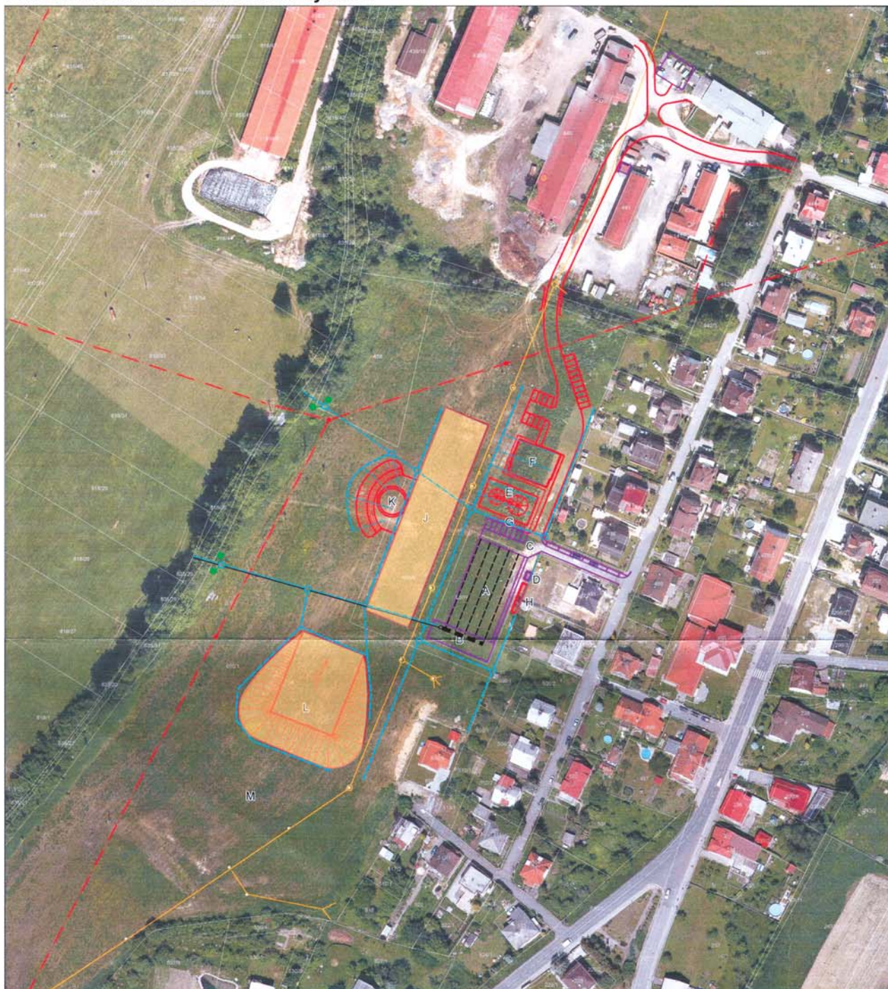
Příloha č.3 Situace odvodňovacího systému
